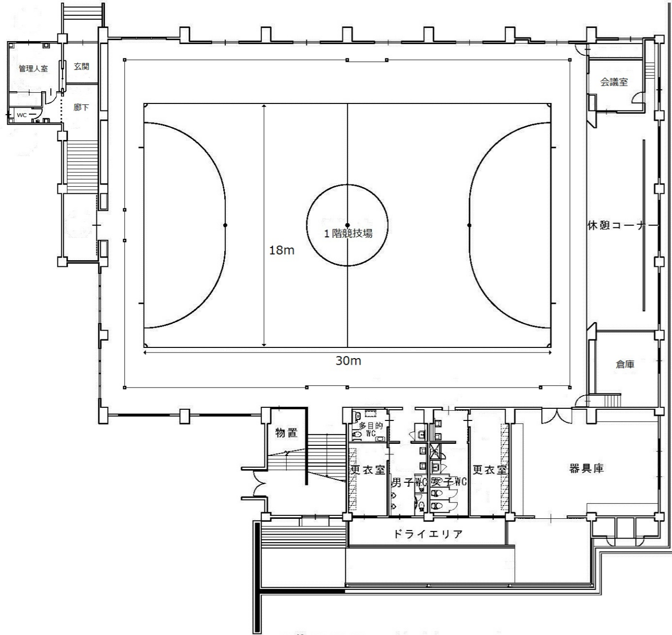
1階平面図
